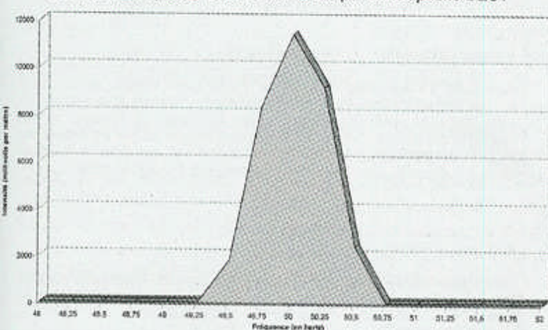
Champ électrique de 48 à 52 hertz émis par un téléphone DECT
